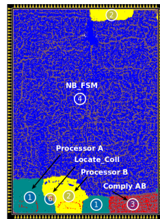
NB Slave ASIC CMOS 28nm FD-SOI layout.
